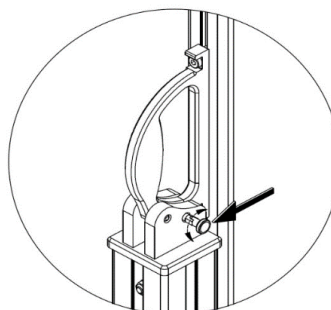
Nakierowanie dolnej części belki przedniej/frontowej na magnes w słupku
