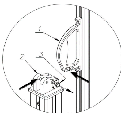
Blokowanie rączki w uchwycie rączki
