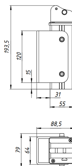
Mocowanie do podłoża naturalnego
